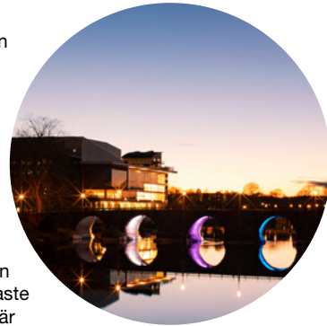
Stenbron i närheten av Gubbholmen
